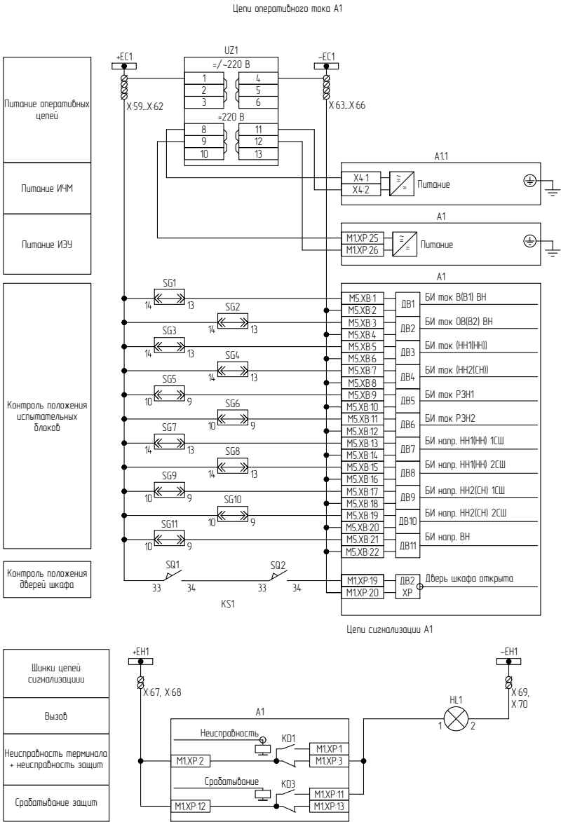
Рисунок Г.2 – Схема электрическая принципиальная (часть 2)
